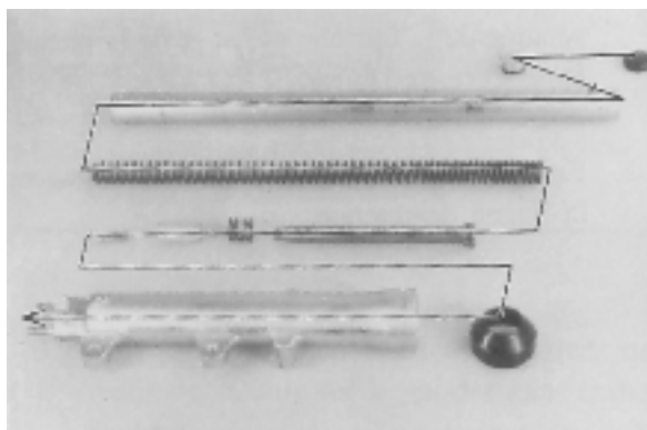
Einzelteile der Vorderradgabel
